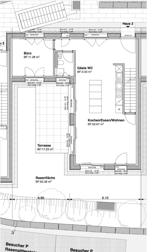
Erdgeschoss
