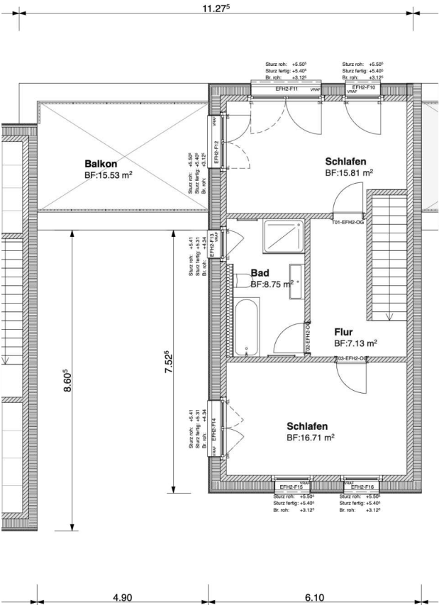
Obergeschoss
