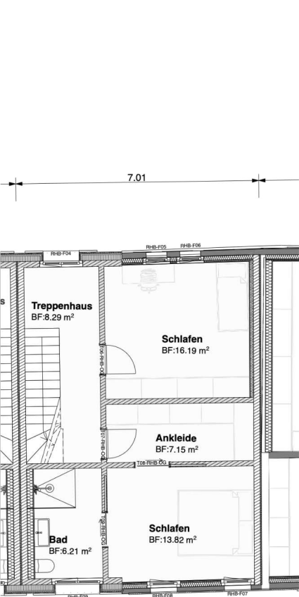
Obergeschoss
