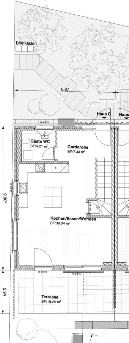
Erdgeschoss
